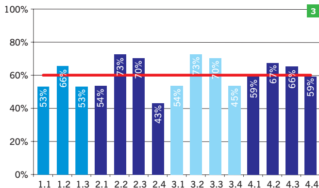
RYS. 3. Projektowe obciążenie cieplne pomieszczeń po termomodernizacji w wariantie 1 jako procent obciążenia początkowego z zaznaczeniem wartości średniej dla budynku wynoszącej 60%;
