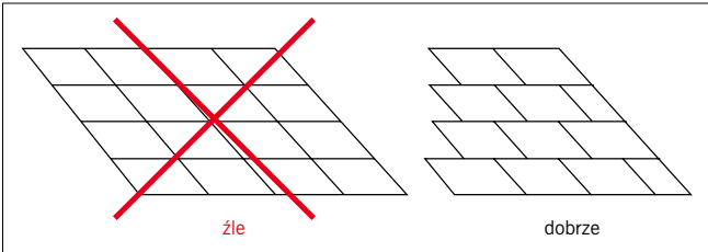
Rys. 5. Układ płyt izolacyjnych układanych na krokwiach Rys. archiwum autora
