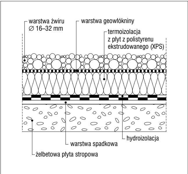
Rys. 2. Stropodach o odwróconej kolejności warstw
