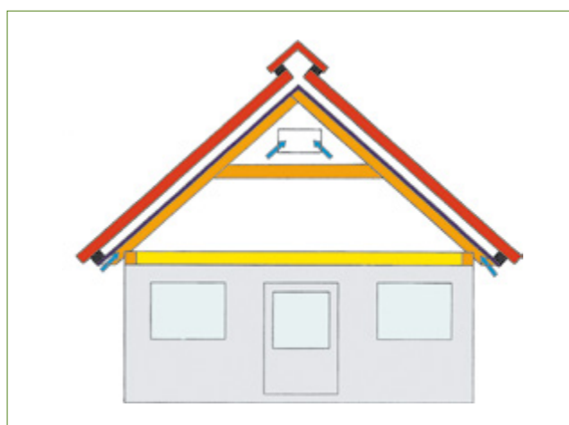
Rys. 3. Typowy dla blachodachówek schemat dachu o poddaszu nieużytkowym bez wentylacji pokrycia zasadniczego – z profilowanymi uszczelkami pod blachą w okapie i pod gąsiorami. W takim dachu warstwą wstępną jest papa lub paroszczelne FWK
