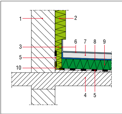
Rys. 3. Wymagania dotyczące izolacyjności cieplnej stropodachów nad pomieszczeniami ogrzewanymi ( t_i > 16^\circ\text{C} ) Rys. archiwum autora
