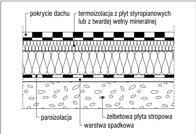
Rys. 1. Stropodach pełny
