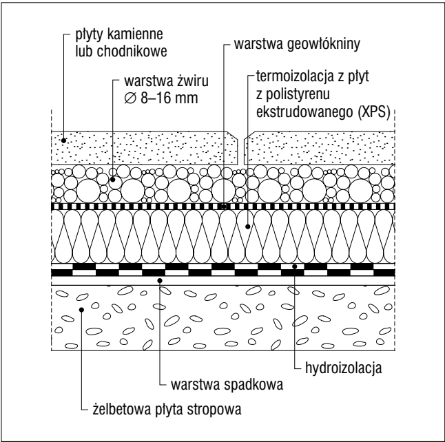
Rys. 3. Stropodach o odwróconej kolejności warstw z nawierzchnią z płyt kamiennych lub chodnikowych
