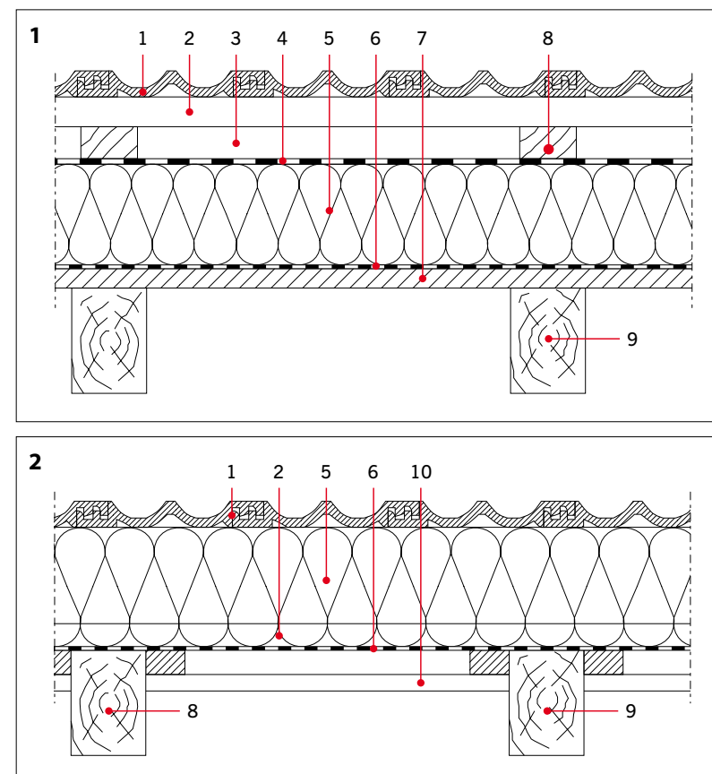
Rys. 1–2. Przekrój przez stropodach z izolacją na krokwiach w dwóch rozwiązaniach: stropodach szczelinowy (1), stropodach pełny (2): 1 – pokrycie dachowe, 2 – łąty, 3 – szczelina wentylowana, 4 – membrana wierzchniego krycia, 5 – izolacja termiczna, 6 – paroizolacja, 7 – deskowanie, 8 – kontrłata, 9 – krokiew dachowa, 10 – płyty gipsowo-kartonowe Rys. archiwum autora
